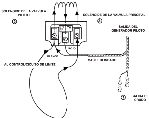
DIAGRAMA MILIVOLTIO PARA VALVULAS MARCA ROBERTSHAW
